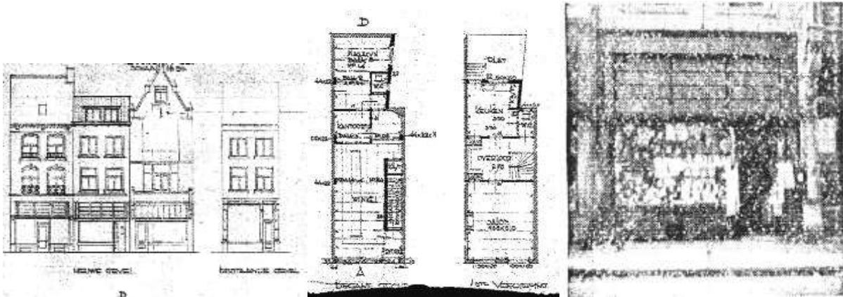
Gevel woning (midden); plattegrond benedenverdieping en eerste verdieping en de enige, helaas zeer vage foto die er is van de winkel, toen die nog van Minco en Lindeman was
